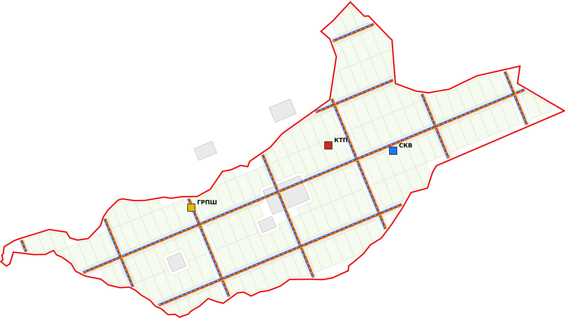
Сводный план инженерных сетей. М 1:2000
